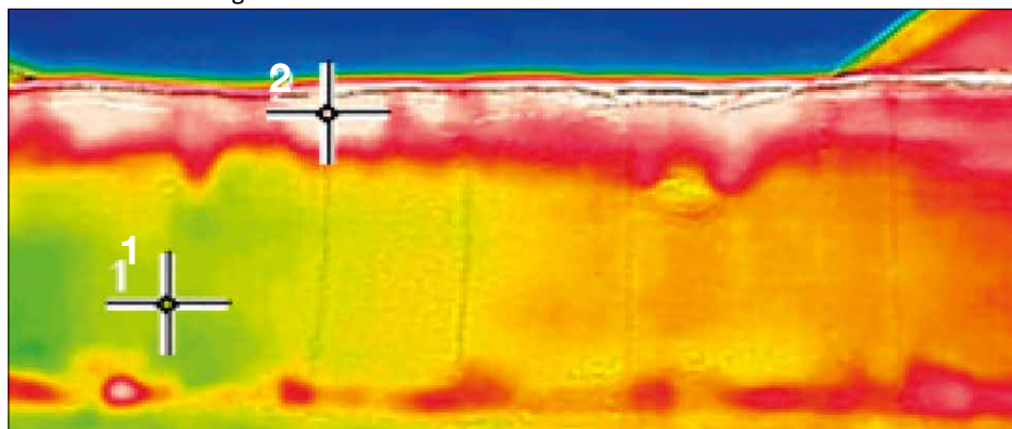
Die Wärmebildkamera zeigt bei einer augenscheinlich gut aussehenden Anschnittfläche deutlich die Nacherwärmung (Messpunkt 1: 17 °C, Messpunkt 2: 29 °C)
